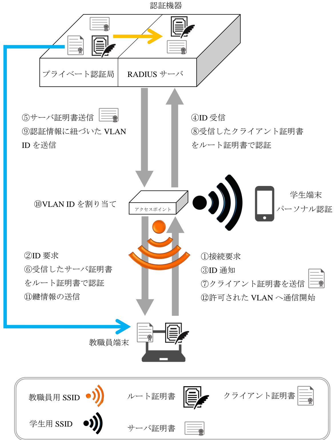
図 2 IEEE802.1X 認証の構成と通信開始までの処理
