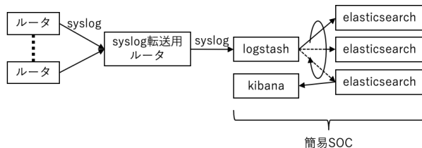
図 2 簡易 SOC への Syslog 転送
