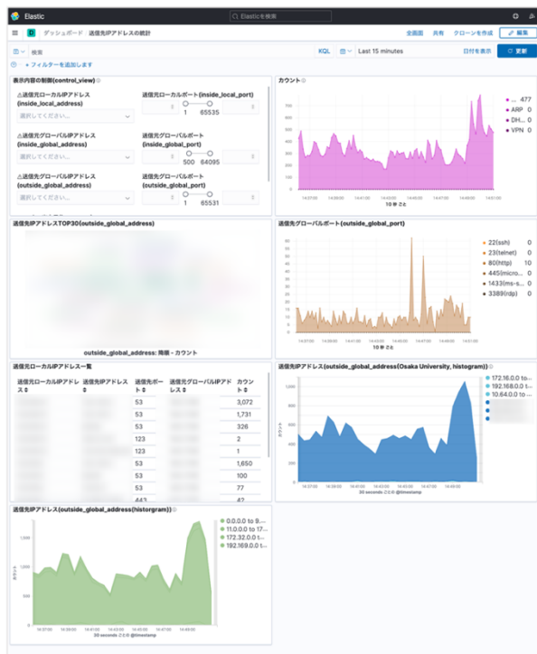
図4 送信先 IP アドレスの統計
